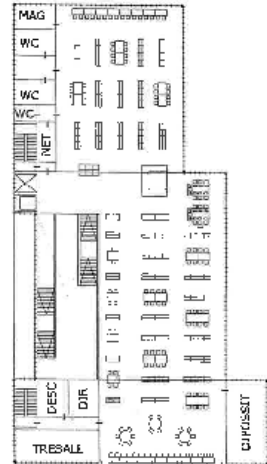
Planta superior
