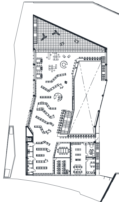
Planta superior
