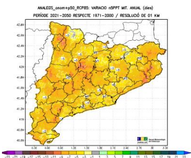
(d) 2021-2050 RCP8.5
