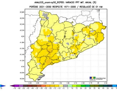
(d) 2021-2050 RCP8.5
