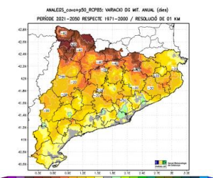
(d) 2021-2050 RCP8.5
