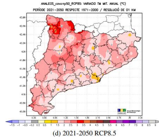
(d) 2021-2050 RCP8.5
