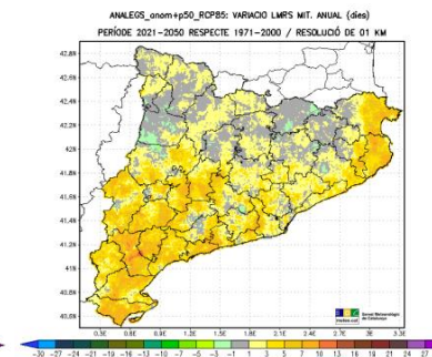
(d) 2021-2050 RCP8.5
