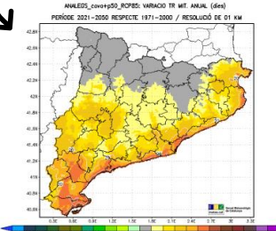
(d) 2021-2050 RCP8.5
