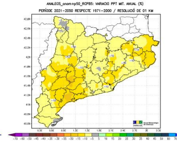
(d) 2021-2050 RCP8.5
