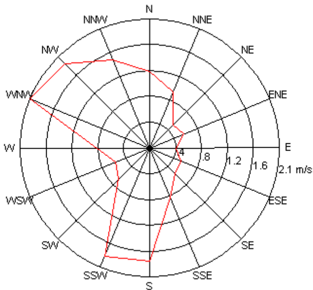
Velocitat del vent - Unitat Mòbil 2 - 14/09/2022 al 21/11/2022
