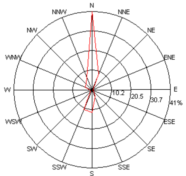
Freqüència del vent - Unitat Mòbil 2 - 14/09/2022 al 21/11/2022
